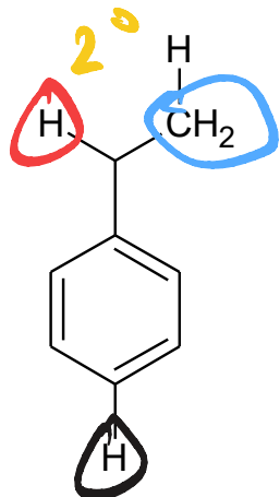
Ethylbenzene
