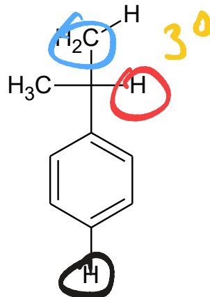
i -Propylbenzene
